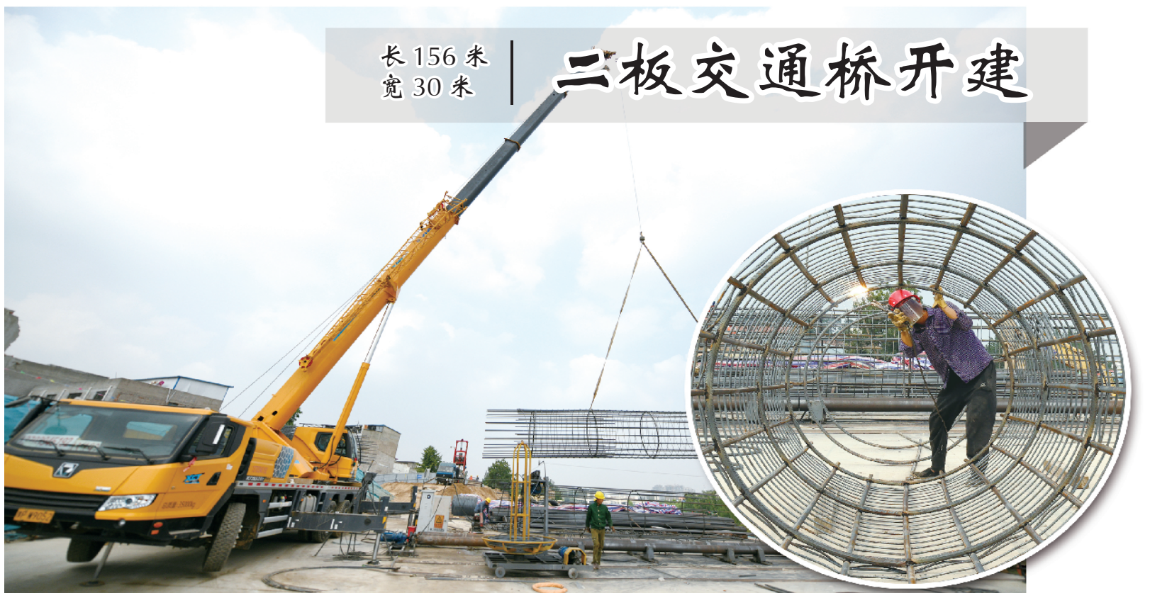
9月14日上午,周口市中心城区坊街西口处贾鲁河岸,各种机械设备正忙碌作业,由河南省水利第二工程局集团有限公司承建的二板交通桥开工建造。据了解,该桥是文昌大道西延横跨贾鲁河的重要工程,桥梁设计全长156米,宽30米,上部采用跨径装配式预应力混凝土先简支后连续箱梁结构,下部采用排架式柱桩结构,预计工期一年。记者 梁照曾 摄 ③19
